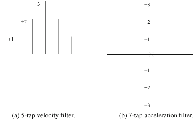
Fig. 13.7 FIR filters
