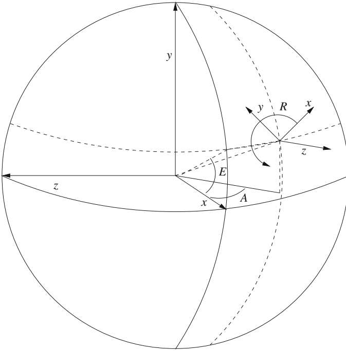
Fig. 7.3 Euler angles
